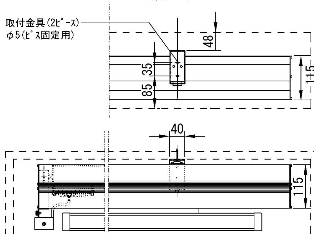
外観図 1/30
