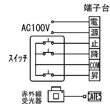
結線図
