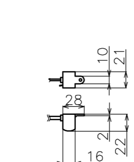
リモコン受光部 S=1/5
