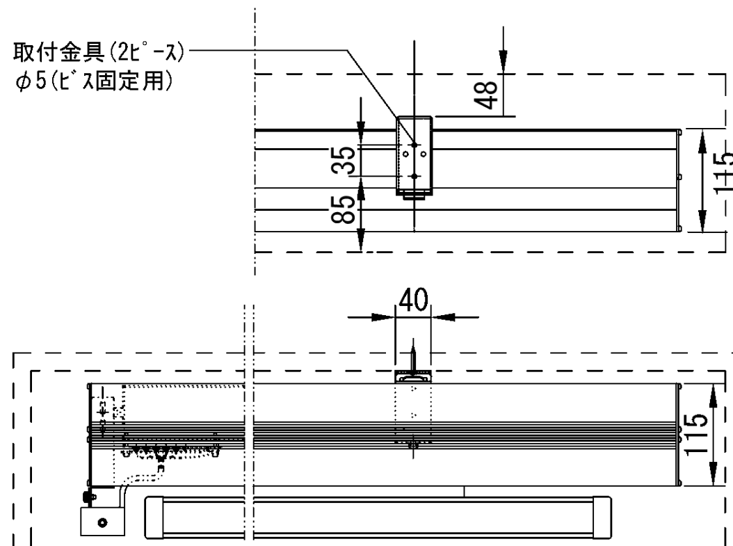
外觀図 1/30
