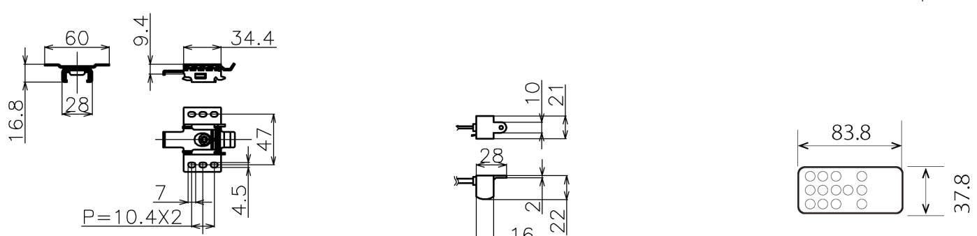
マウントブラケット S=1/5 リモコン受光部 S=1/5 リモコン
