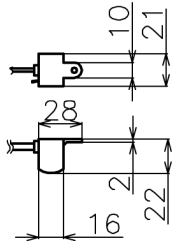
リモコン受光部 S=1/5
