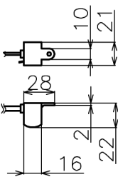
リモコン受光部 S=1/5
