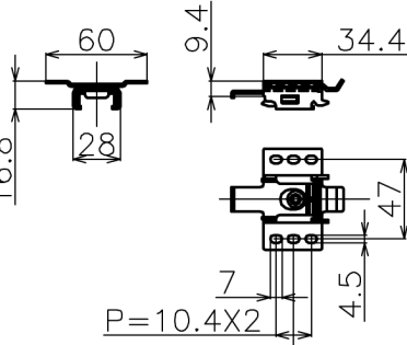
マウントブラケット S=1/5
