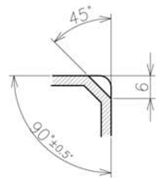
補強用リブ詳細 尺度1:1
