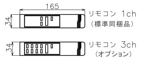
リモコン送信機 S=1/5
