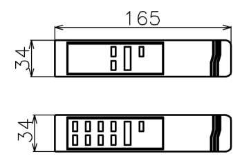
リモコン送信機 S=1/5
